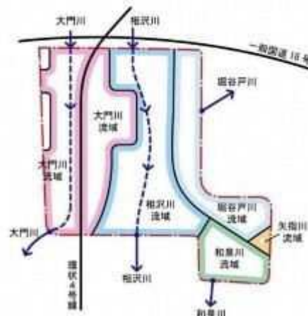
図 2.2-4 流域の状況
