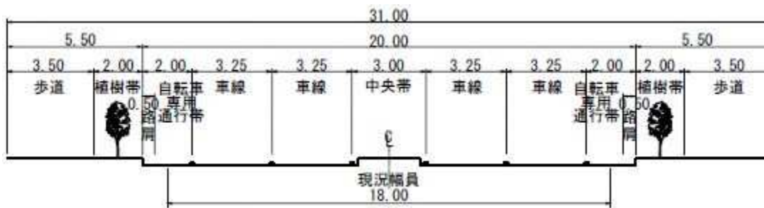
図 2.2-2(2) 環状 4 号線 (南区間) の標準断面図
